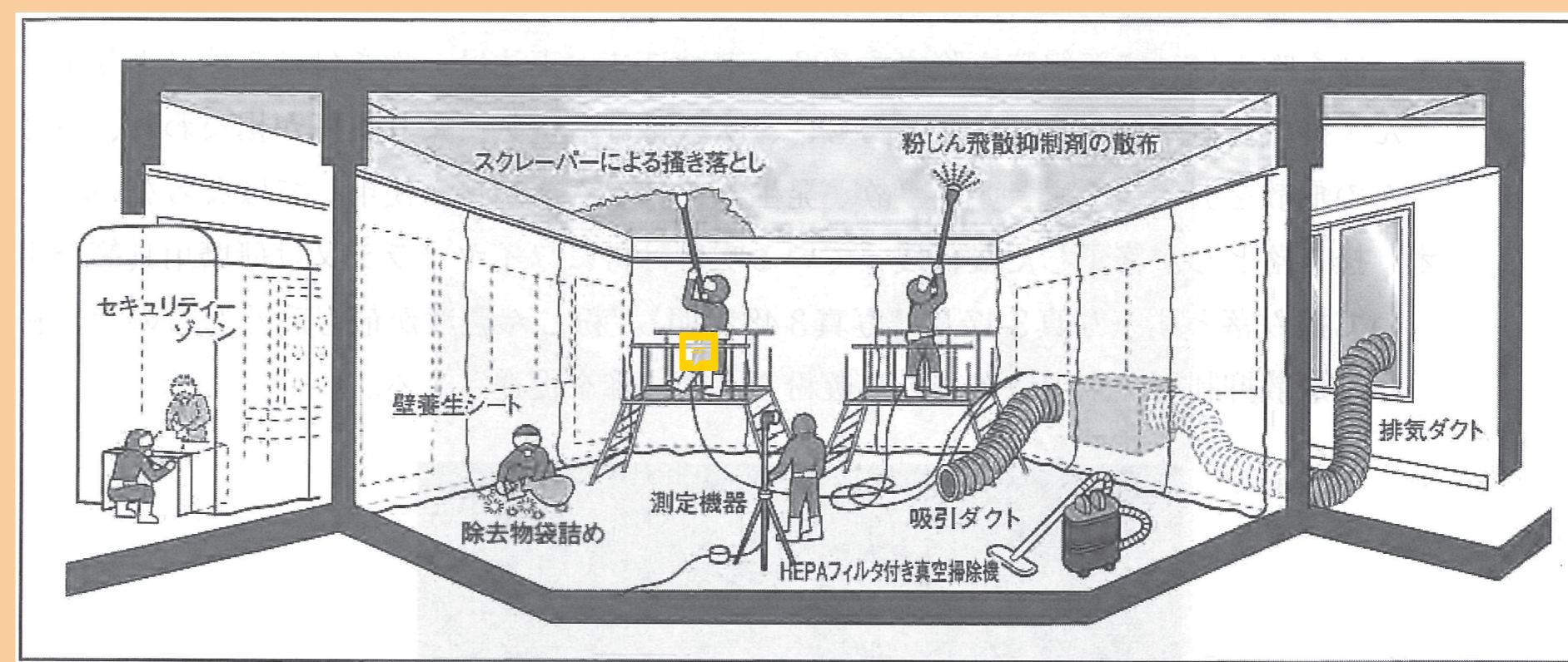
石綿含有吹付け材除去作業概念図
